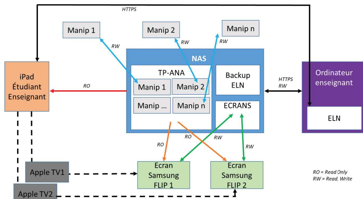
Figure 1. Architecture réseau et fonctionnalités envisagées
